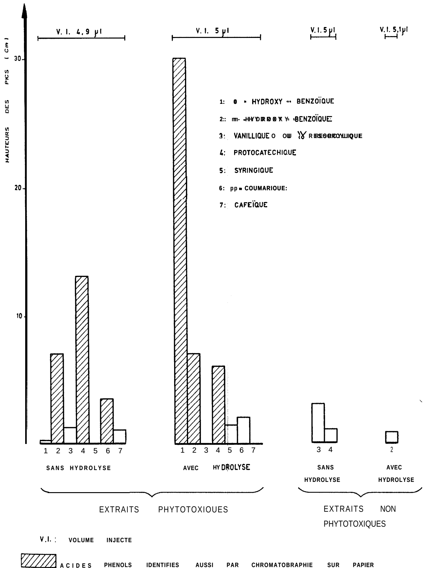
FIGURE 4. - IDENTIFICATION PAR CHROMATOGRAPHIE EN PHASE GAZEUSE, DES ACIDES PHENOLS CONTENUS DANS LES EXTRAITS PHYTOTOXIQUES ET NON PHYTOTOXIQUES OBTENUS APRES HYDROLYSE ACIDE OU SANS HYDROLYSE, A PARTIR D'UNE EXTRACTION A L'ETHANOL FAITE SUR DES RACINES DE CORYD.
