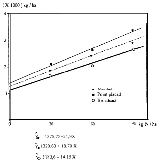
Figure 1 : Réponse du maïs à l'urée en fonction des méthodes d'application - Nioro 1987
