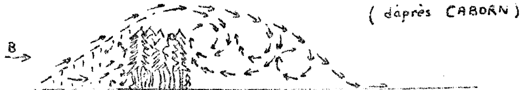
Flux du vent à travers un rideau protecteur A: moyennement perméable B: dense
