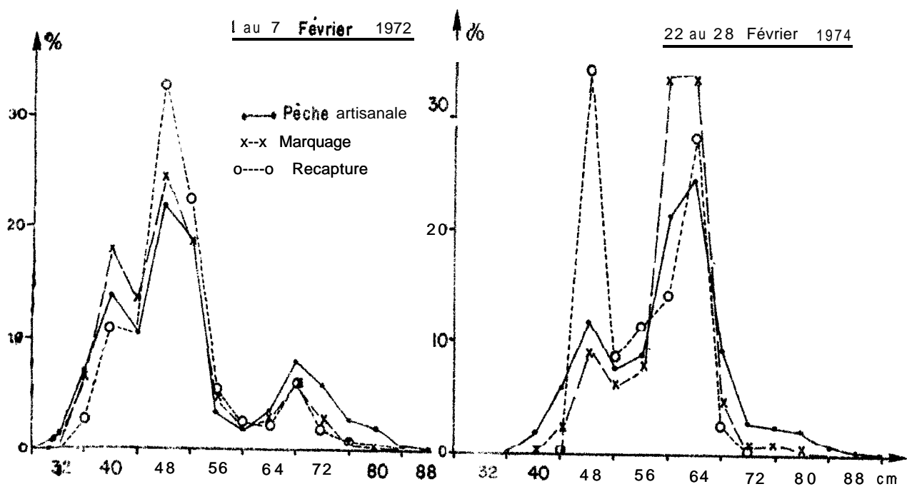
Fig. 4 - Distributions de fréquence de tailles de poissons marqués, des poissons recapturés et de la population exploitée par la pêche artisanale à CAYAR.
