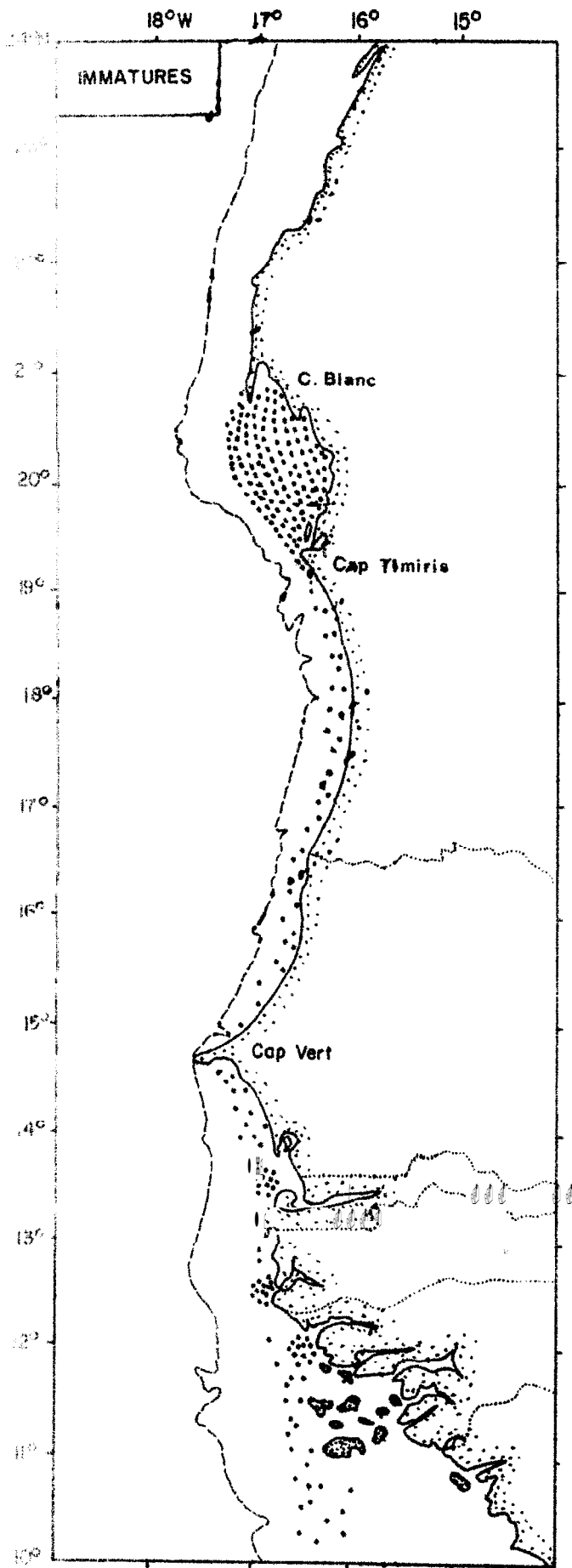
Fig. 5 - Cycle biologique de tassergol
