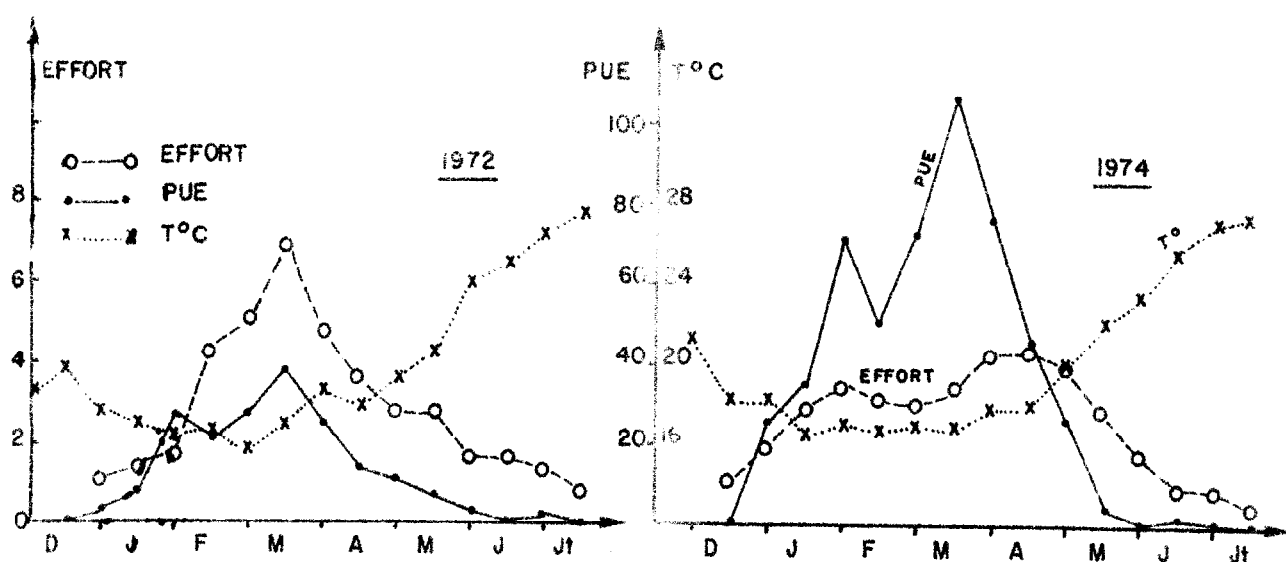
Fig. 3 - Effort (milliers de sorties de pirogues), PUE (nombre poissons par pirogue) et température de surface par quinzaine à CAYAR en 1972 et 1974.
