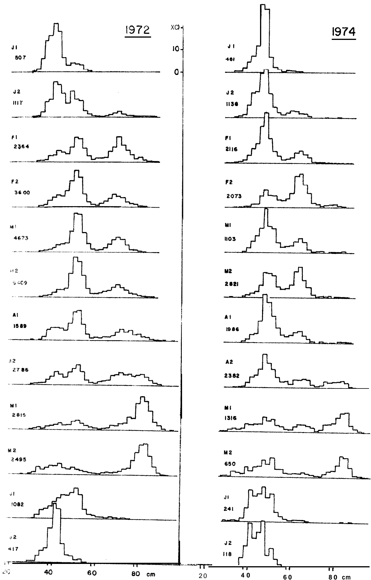
Fig. 2 - Distributions de fréquence de tailles bimensuelles des tassergals débarqués à CAYAR en 1972 et 1974.
