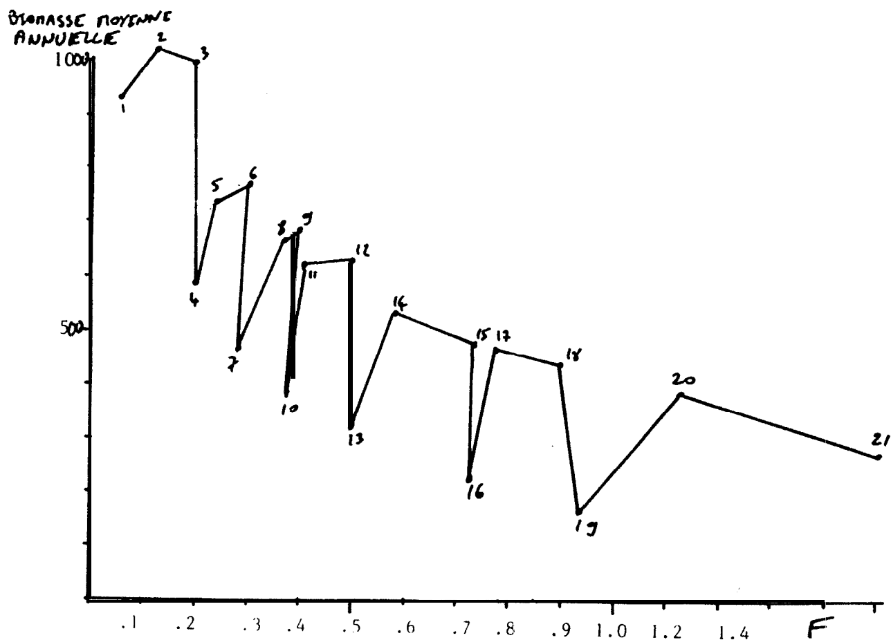
Fig. 6b.- Biomasse et taux de mortalité par pêche avec simulation d'un stock à capturabilité constante, recrutement mensuel variable (figure 2) et effort de pêche variable selon la pue.
