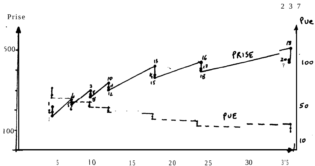
Fig. 1a.- Relation prises, pue, effort avec simulation à recrutement et capturabilité constants. Chaque point correspond à la prise/pue et l'effort d'une année de pêche,
