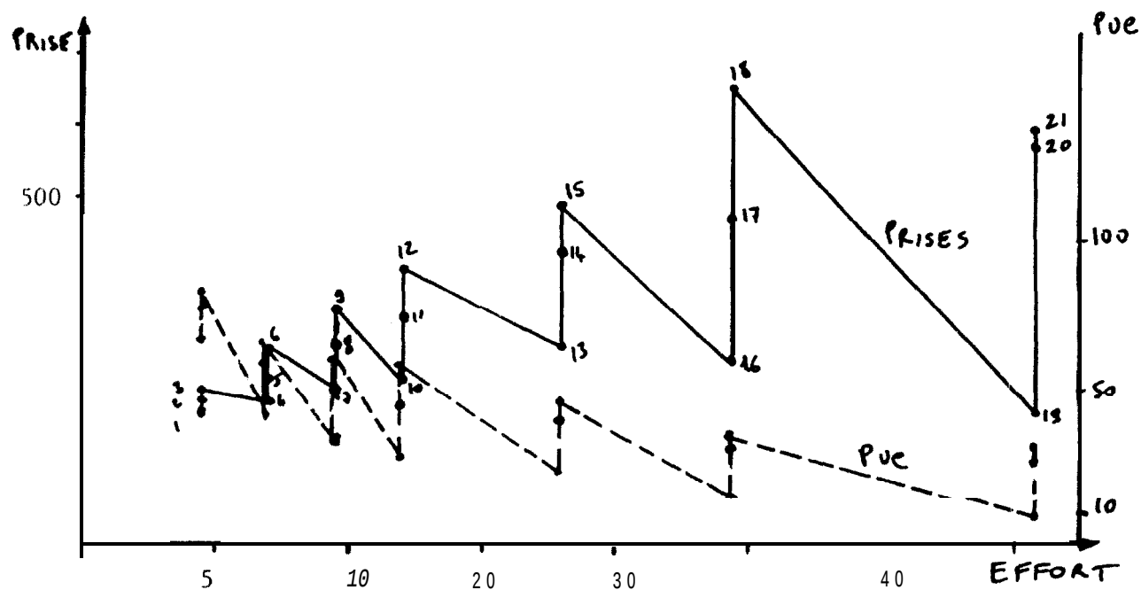
Fig. 3a.- Prises, pue et efforts de pêche annuels avec simulation d'un stock à capturabilité constante et recrutement variable mensuellement selon le schéma de la figure 2. (Chaque point représente une année de pêche, numérotées de 1 à 21). Les courbes A et B tracées à l'oeil traduisent le type de la production en fonction de l'effort qui semblent exister en périodes de forts recrutements (courbe A) ou de faibles recrutements (courbe B).
