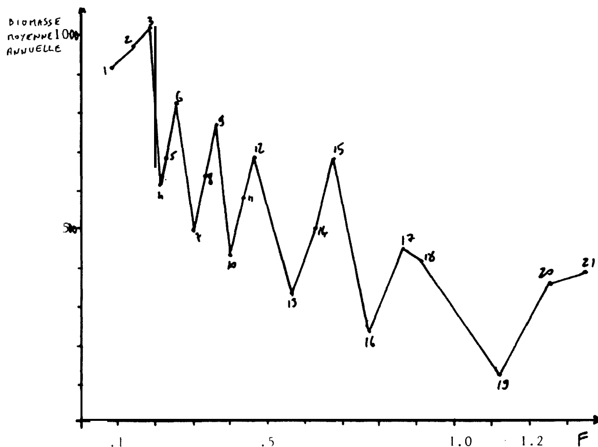
Fig. 3b.- Biomasse et taux de mortalité par pêche avec simulation d'un stock à capturabilité constante et recrutement variable selon le schéma de la figure 2.
