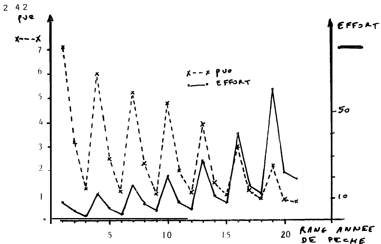
Fig. 7.- p u e annuelles du stock simulé à capturabilité variable (§ 5) et efforts de pêche variables selon le niveau de la pue, calculés à partir de ces p u e pour le stock décrit au § 7.
