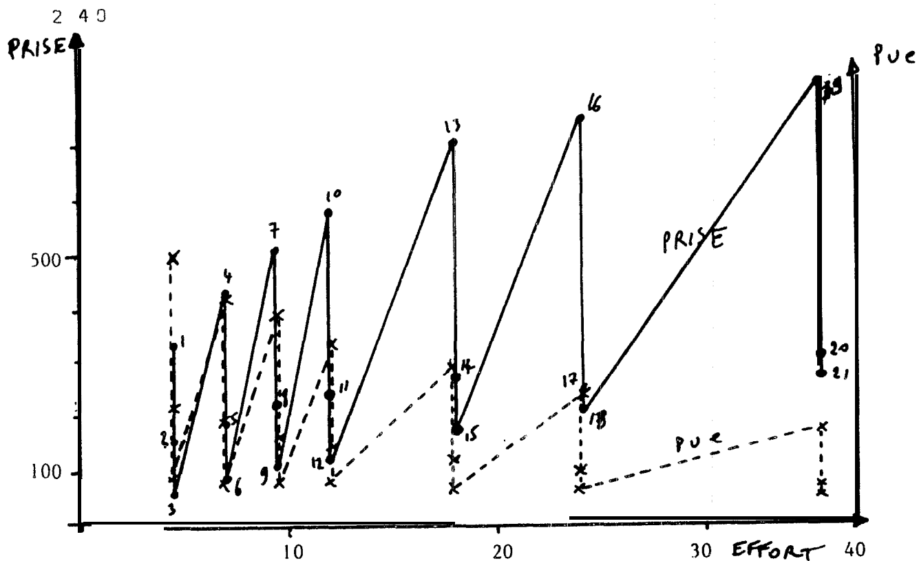
Fig. 5a. - Relation prise, pue, effort avec simulation d'un stock à recrutement constant et- capturabilité variable mensuellement selon le schéma de la figure 4.
