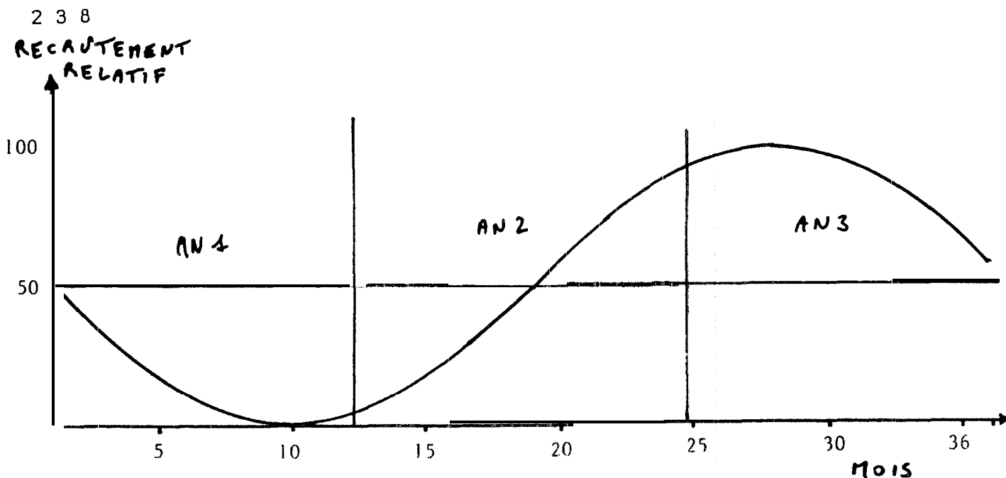
Fig. 2.- Variation5 du recrutement mensuel dans les pêcheries n° 2 et exploitant un stock à recrutement variable.
