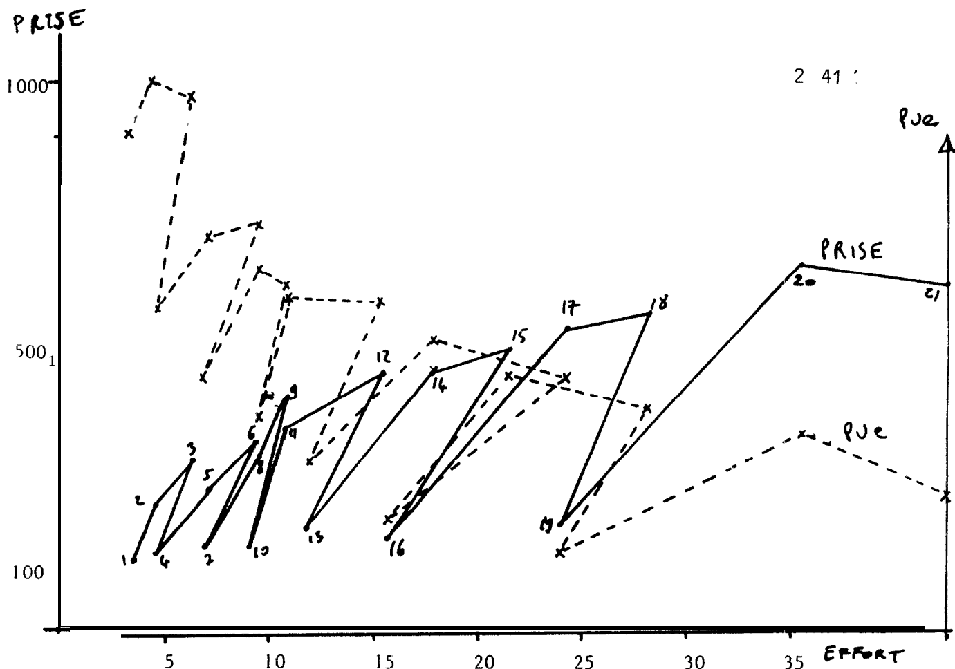
Fig. 6a.- Prises, pue et efforts de pêche annuels avec simulation d'un stock à capturabilité constante, recrutement mensuel variable et effort mensuel variable selon la pue.
