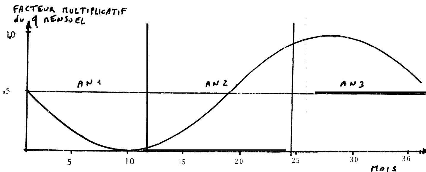
Fig. 4 - Variations du facteur q mensuel (capturabilité) dans la pêche de 1 'exemple n° 1 et exploitant un stock à capturabilité variable.
