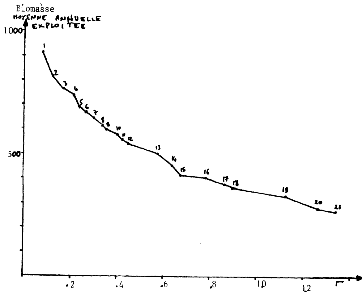
Fig. 1b.- Relation biomasse et mortalité par pêche avec une simulation à recrutement et capturabilité constants.
