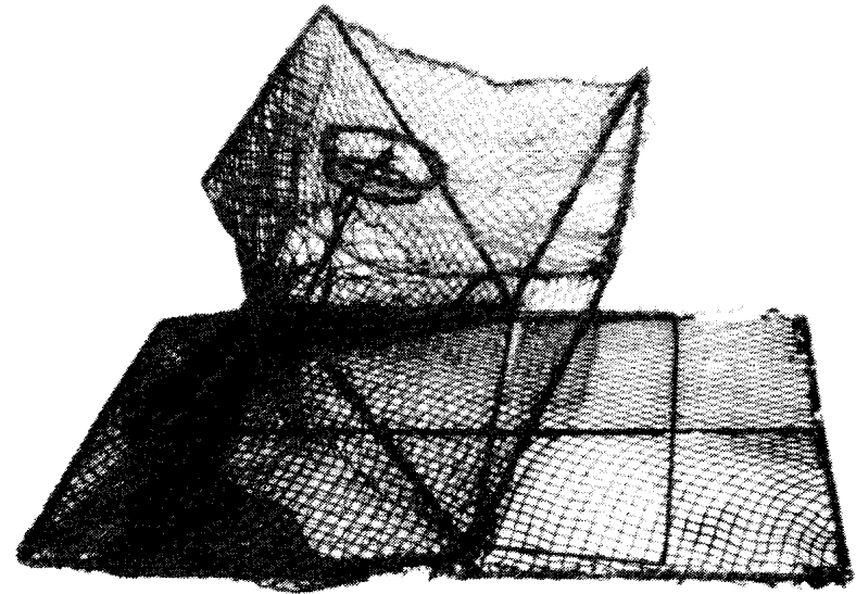
Photo 3 : Nouveau casier à moitié plié
