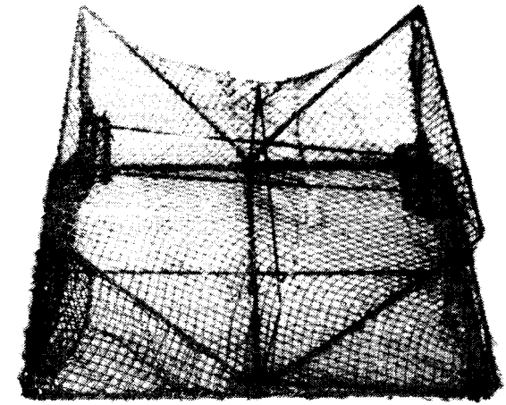
Photo 2 : Nouveau casier déplié
