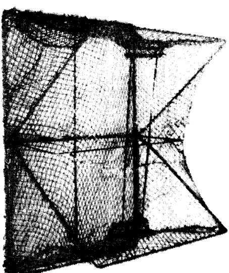
Photo 7 : Nouveau casier déplié
