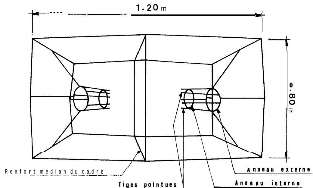
Fig. 2-SCHEMA DU NOUVEAU CASIER PLIABLE
