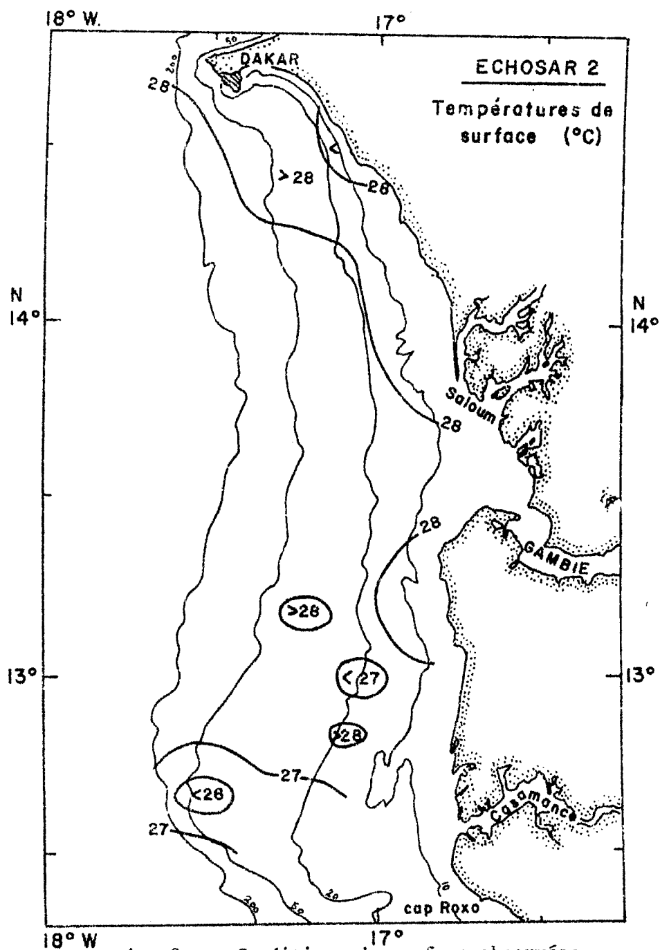
Fig. 8 a.- Conditions de surface observées en septembre 1980 au cap Vert. Température.
