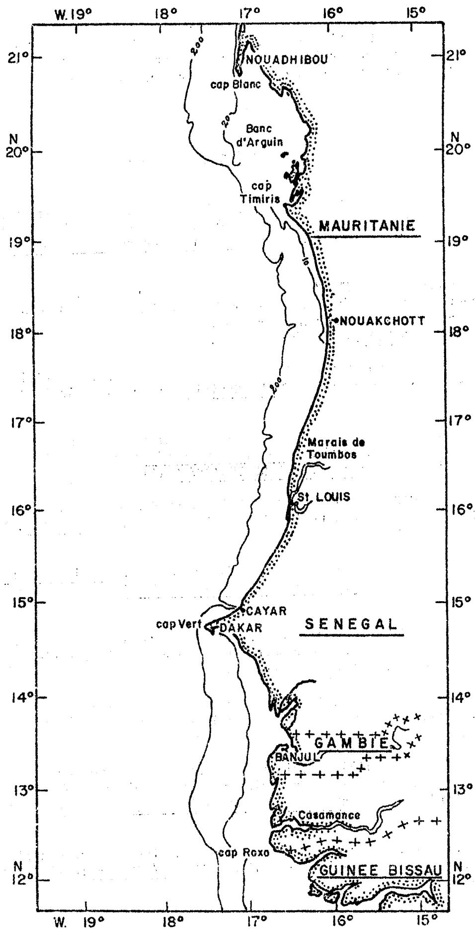
Fig. 1 : Extension de la zone étudiée.
