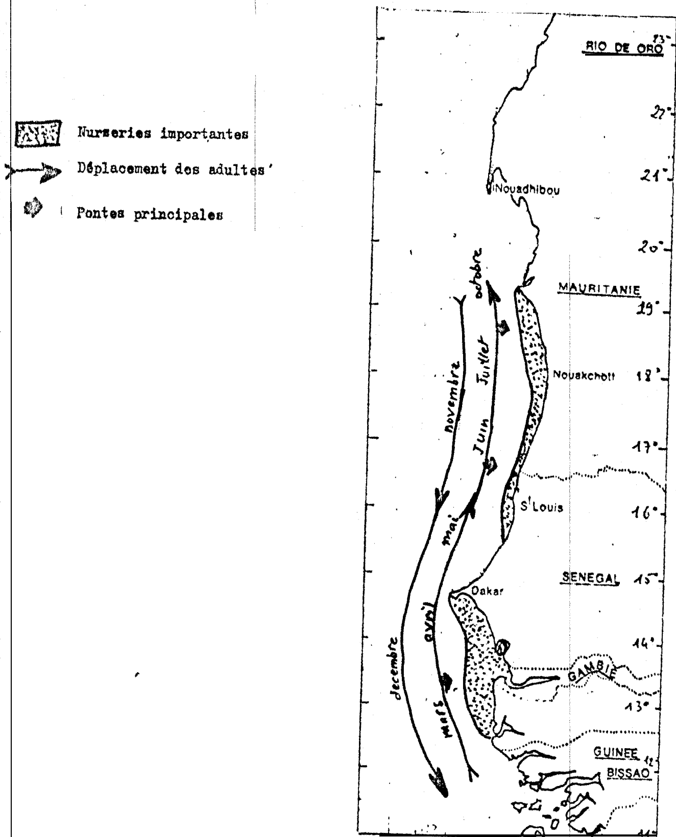
Fig.41-Cycle migratoire, périodes de ponte, nurseries et localisation des principales concentrations d'adultes de Caranx rhonchus dans la zone sénégalo-mauritanienne
