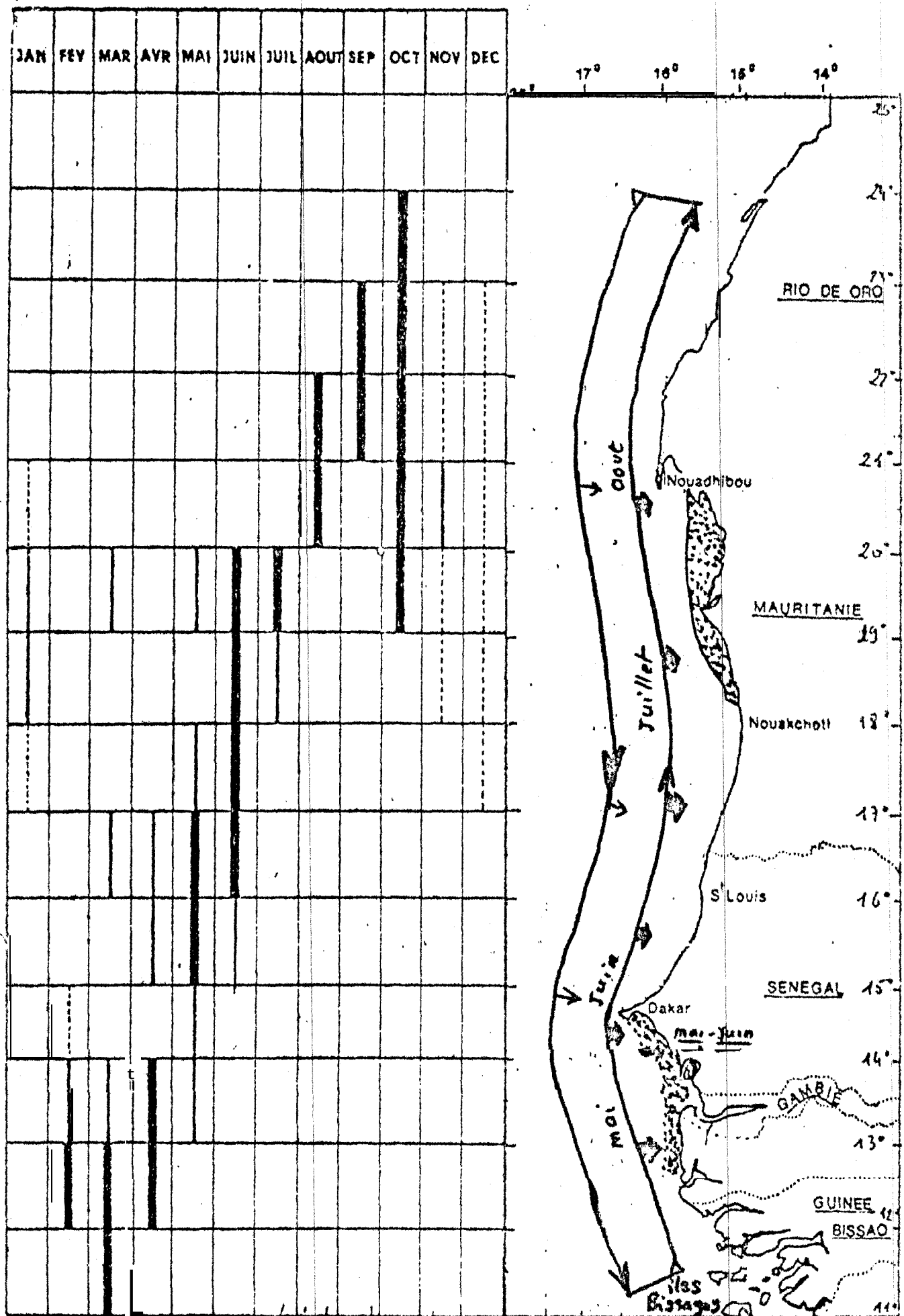
Fig. 38 Cycle migratoire, périodes de ponte, nurseries et localisation mensuelle des principales concentrations d'adultes de Sardinella aurita dans la zone sénégal-mauritanienne
