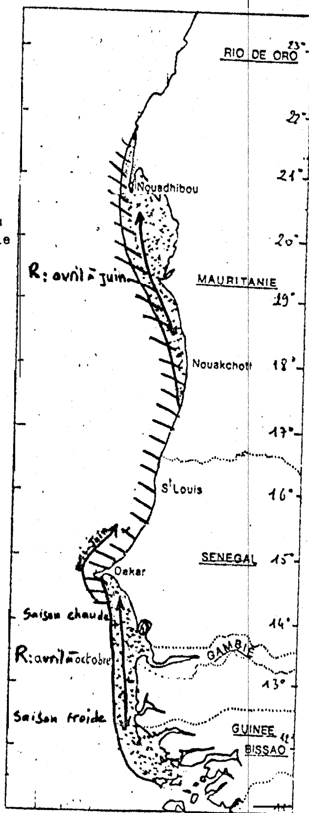
Fig. 40 - Déplacements, principales périodes de reproduction et nurseries de Sardinella maderensis dans la zone sénégal-mauritanienne
