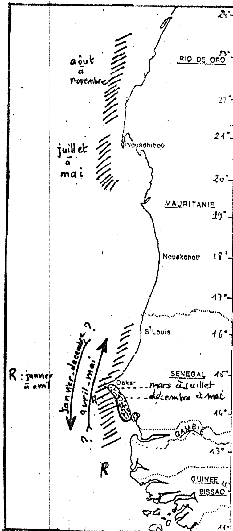
Fig.44-Déplacements probables de principales zones de concentration et de reproduction de Scomber japonicus dans la zona sénégal-mauritanienne
